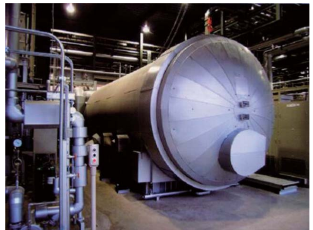
愛知万博 NEDO 館1階に設置された MCFC (Vol. 5-1) (提供: NEDO)
